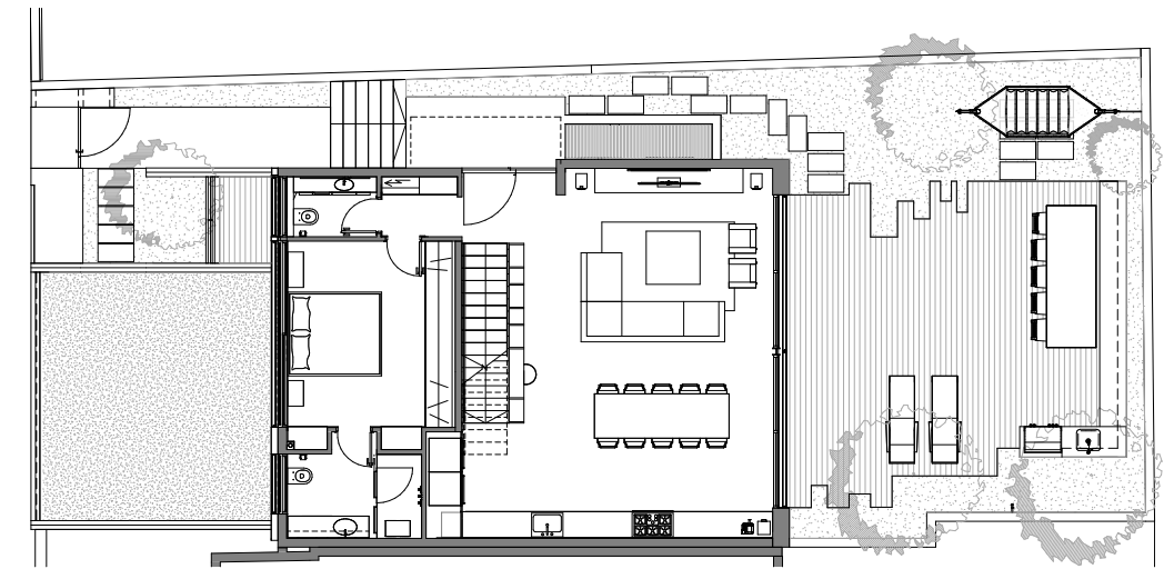
קומת כניסה
