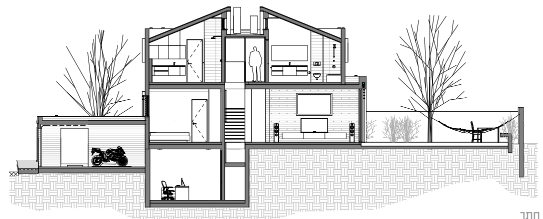
חתך
